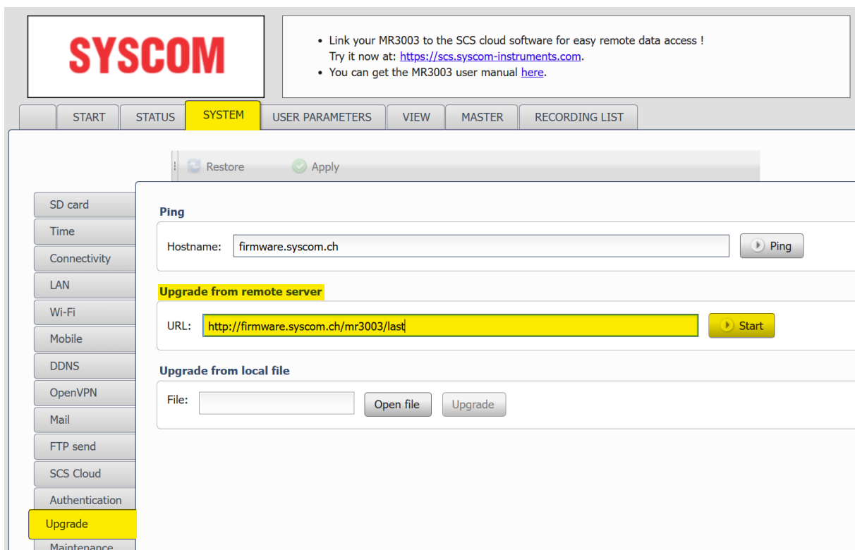
Abb. 5: Eingefügter URL-Link
