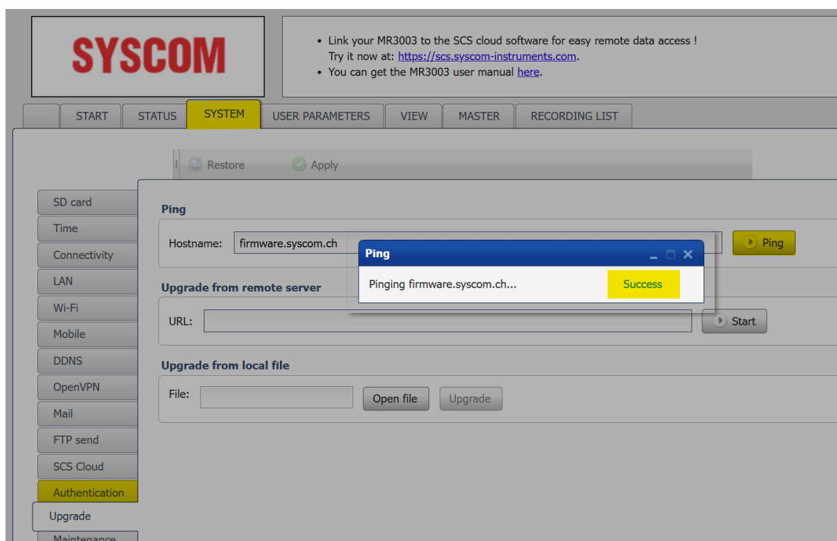
Abb. 4: Erfolgreiche Internetverbindung
